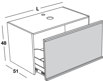
Waschtischunterschrank mit einer großen Schublade für Aufsatzwaschbecken. Washbasin base unit with one big drawer for sit-on washbasin.
