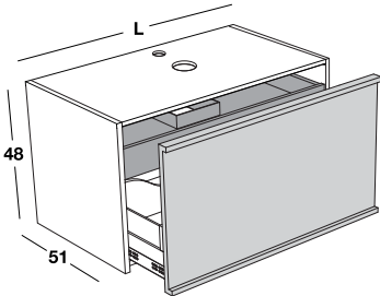
Waschtischunterschrank mit einer großen Schublade und internem Schubfach für Aufsatzbecken. Washbasin base unit with one big drawer and internal drawer for sit-on washbasin
