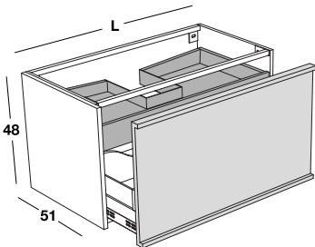
Waschtischunterschrank mit einer großen Schublade und internem Schubfach. Washbasin base unit with one big drawer and internal drawer.
