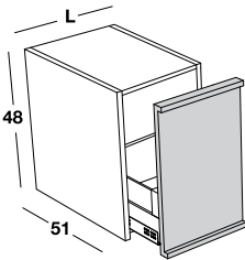
Möbel mit einer Schublade. Base unit with 1 drawer.
