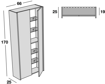
Hochschrank 2 Holztüren, 4 Glasregale und 1 festes Regal, Tiefe 19 cm Column 2 wooden doors, 4 glass shelves and 1 fixed shelf depth 19 cm
