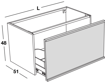
Waschtischunterschrank mit einer großen Schublade. Washbasin base unit with one big drawer.
